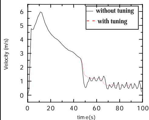
Fig. 27. Velocity Profiles.
